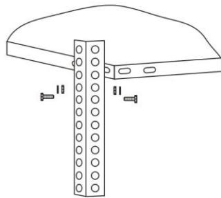
2. Узел крепления средних полок
