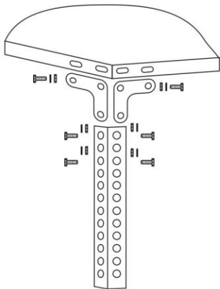
1. Узел крепления верхней и нижней полки
