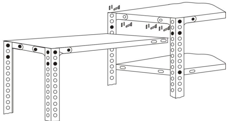
3. Порядок сборки стеллажей в "ленту"
